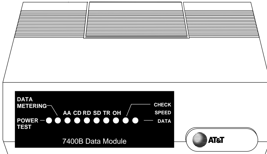
FIGURE 5-2. The 7400B Plus Data Module
